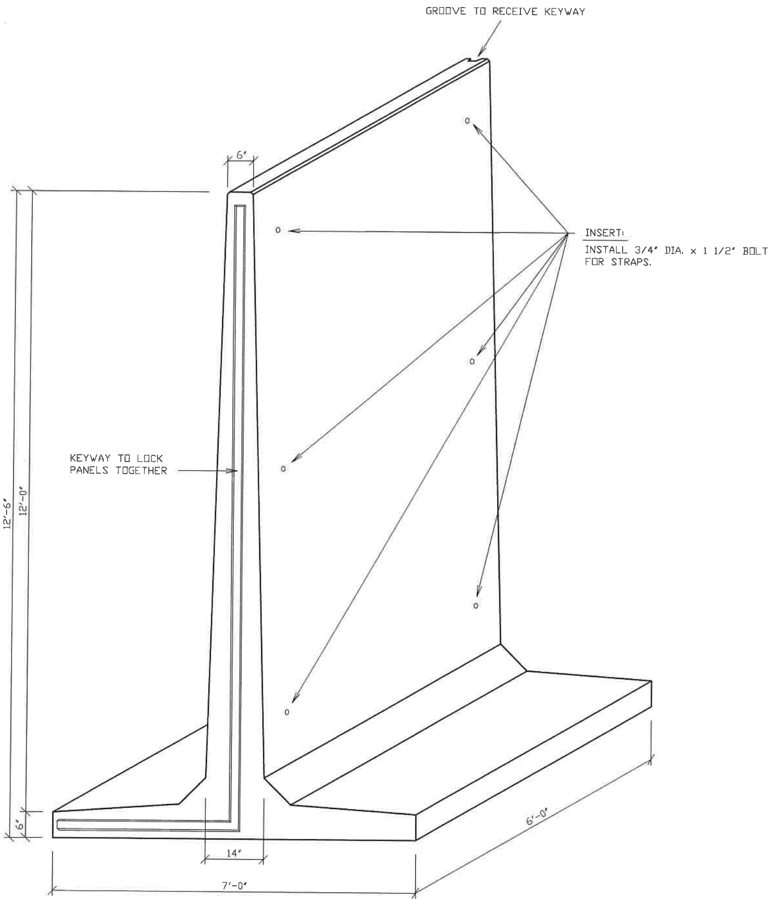
STANDARD 12'-6" PRECAST UNIT N.T.S.
